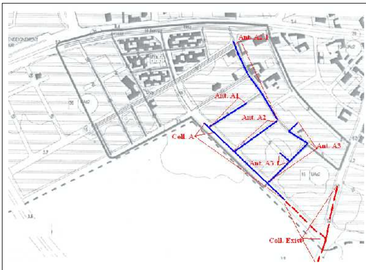
Figure 3 : Plan de situation des collecteurs d'assainissement à exécuter
