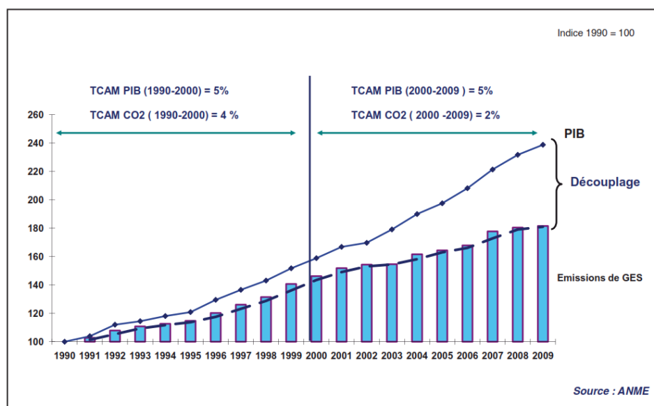
Figure 6. Croissance économique et émissions de GES dues à l'énergie
